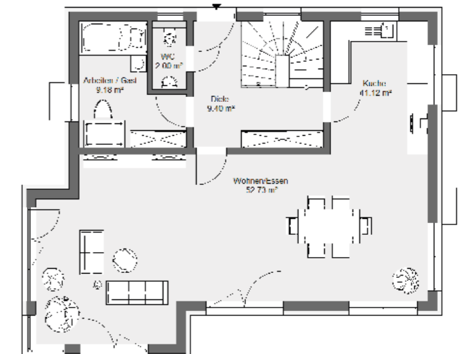
Erdgeschossvariante / Haus mit Keller
