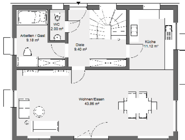
Erdgeschossvariante mit Keller
