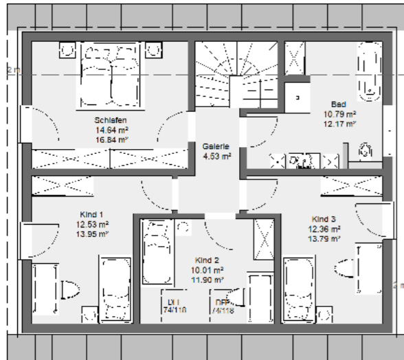
Dachgeschossvariante mit drei Kinderzimmer
