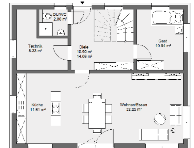
Erdgeschossvariante ohne Keller
