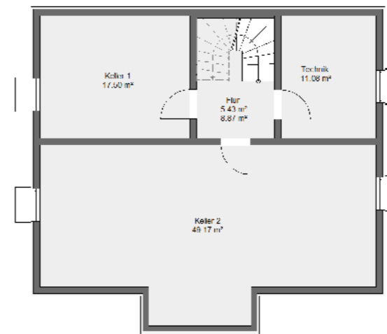
Kellergeschoss
