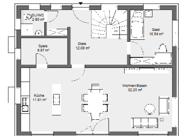
Erdgeschossvariante / Haus mit Keller
