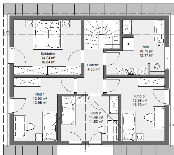
Obergeschossvariante EG wie Basishaus
