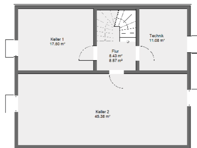
Kellergeschoss
