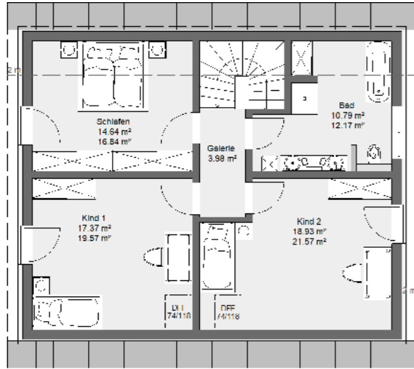
Dachgeschossvariante mit zwei Kinderzimmer
