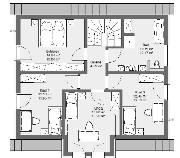
Dachgeschossvariante
