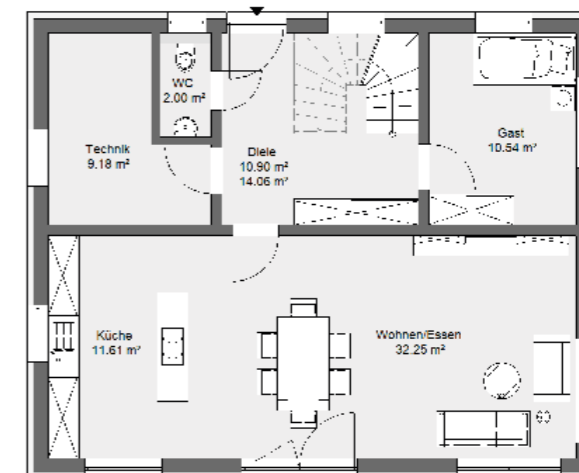
Erdgeschossvariante / Haus ohne Keller
