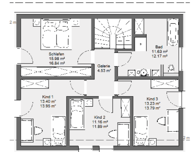
Dachgeschossvariante EG wie Basishaus
